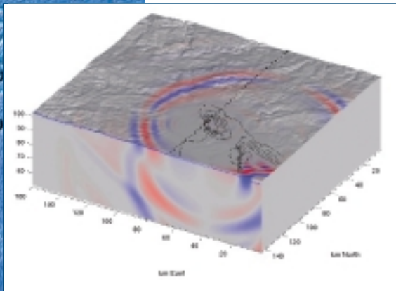
Schnappschuss einer Erdbebenwellenausbreitung im Kölner Becken. Die Blickrichtung ist nach Süd-Osten. In der rechten unteren Bildecke sind verstärkte Effekte zu erkennen, die durch die dort vorliegende Sedimentstruktur bedingt sind.
