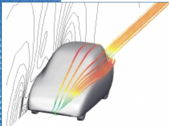
Visualisierung der Strömung um ein PKW-Modell im Windkanal.
