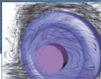
Simulation einer turbulenten Luftströmung im Inneren eines Radkastens. Direkte Volumenvisualisierung mittels 3D Line Integral Convolution (LIC).
