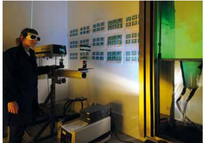
Beurteilung der Mischungsqualität eines Vormischbrenners im Wasserkanal durch laserinduzierte Fluoreszenz (Quelle: Lehrstuhl für Thermodynamik TU München)
