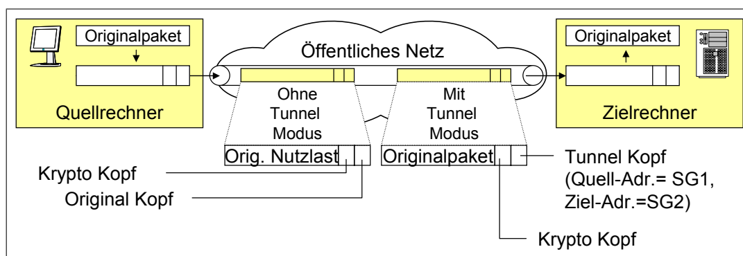
Abbildung 4: Ende-zu-Ende VPN
