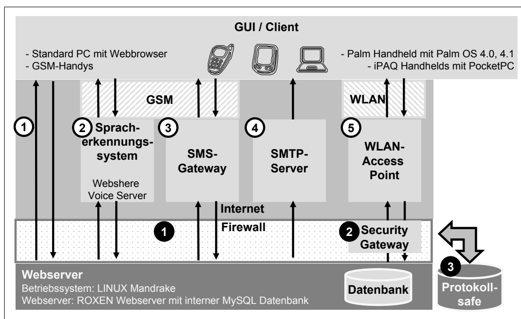
Abbildung 5: Abgesicherte Systemarchitektur von U-Know
