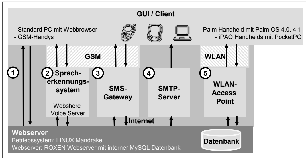
Abbildung 3: Systemarchitektur von U-Know
